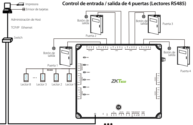
Control de entrada / salida de 4 puertas (Lectores RS485)
