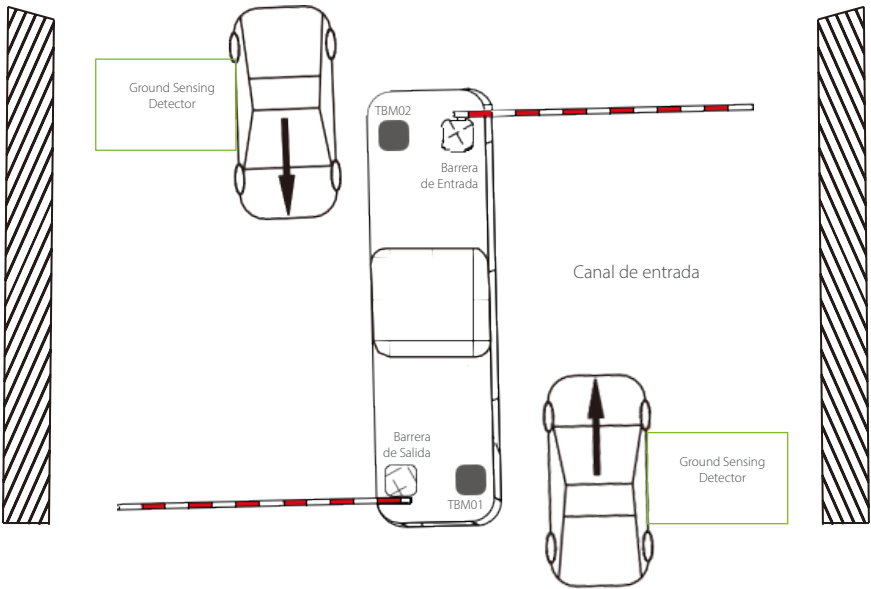
Diagrama de especificaciones de instalación de sensores de detección
